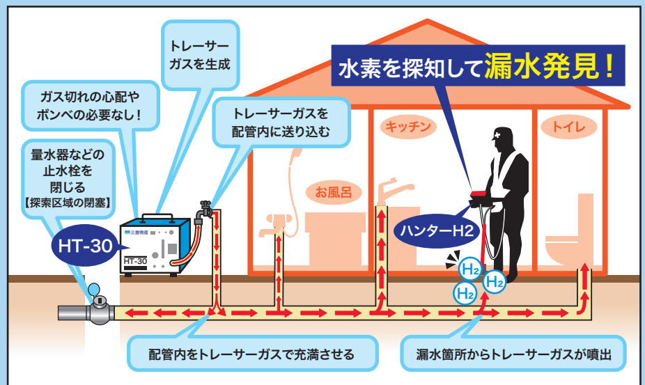
▲水素ガス造成装置ハイドロ トレーサーHT-30
